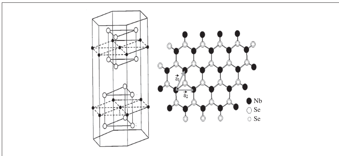
Рис. 1. Фрагменты кристаллической структуры диселенида ниобия (слева) и его молекулярного монослоя (справа). Атомы Se расположены над – и под сеткой атомов Nb. a_1 , a_2 – базисные вектора гексагональной сетки атомов ниобия.
