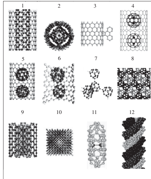
Рис. 6. Атомные модели некоторых предложенных нами новых нанокompозитов: 1 – нанокабель C-НТ@BN-НТ; 2 – нанокабель Fe_n@C -НТ; 3 – углеродная нанотрубка (C-НТ), функционализированная ковалентно-связанными графитовыми пластинками; 4 – пипод Ti_2@C_{80}@C -НТ; 5 – пипод C_{60}@BN -НТ; 6 – пипод V_{12}C_{12}@BN -НТ; 7 – гипералмаз C_{28} ; 8 – автоинтеркалированный гипералмаз C_{28} ; 9 – нанокабель Co_m@C -НТ; 10 – алмазоподобное нановолокно BN в графитоподобной «оболочке»; 11 – углеродный sp^2 + sp^3 «нанобатон»; 12 – углеродная нанотрубка, функционализированная ДНК.
